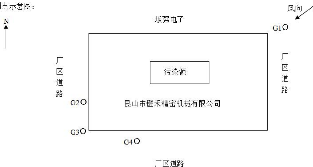
图 7.1-1 本项目废气监测点位示意图
