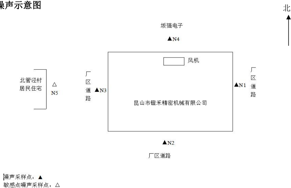
图 7.1-2 本项目噪声监测点位示意图
