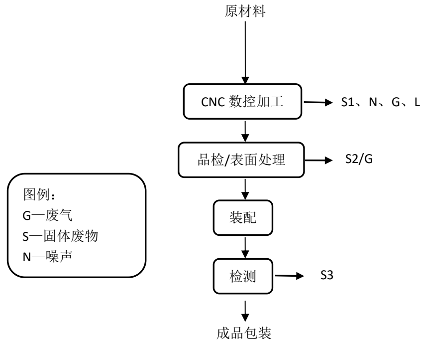
图 3.5-1 产品生产工艺流程图
