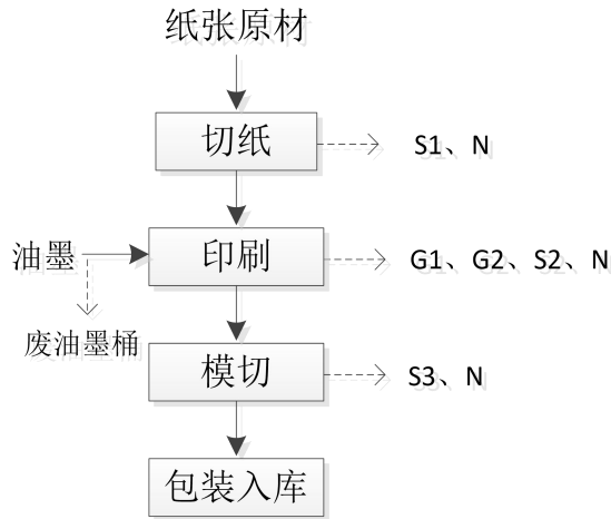
图 3.5-1 项目生产工艺流程图
