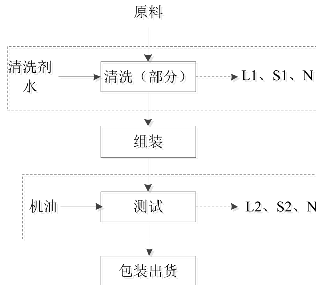
图 3.5-1 生产工艺流程图（虚线框内为本次技改新增工艺）
