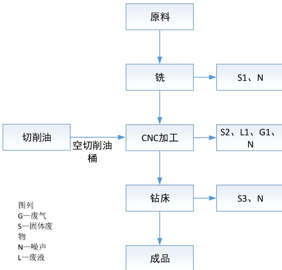
图 3.5-1 项目生产工艺流程图
