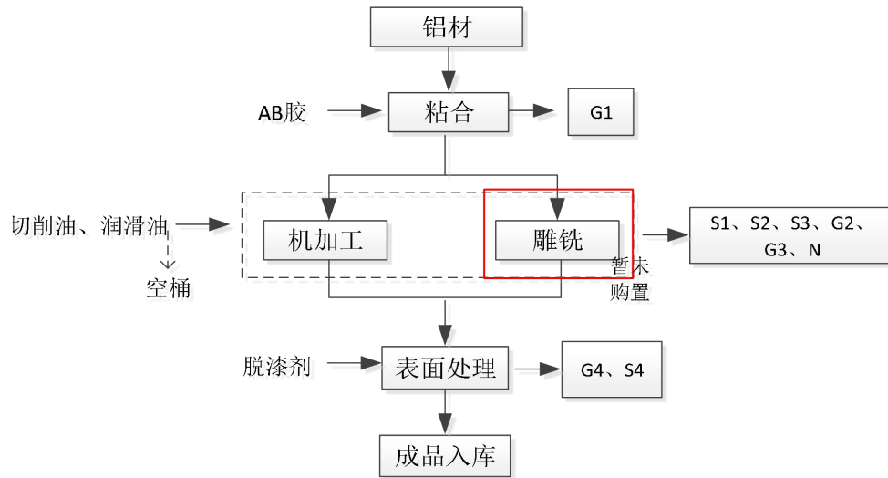
图 3.5-1 生产工艺及产污环节图
