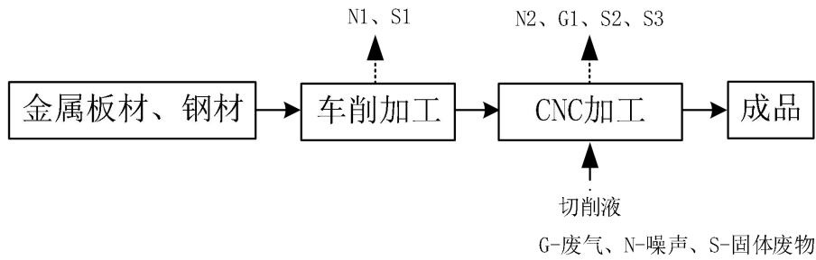
图 3.5-1 法兰件生产工艺流程及产污环节图
