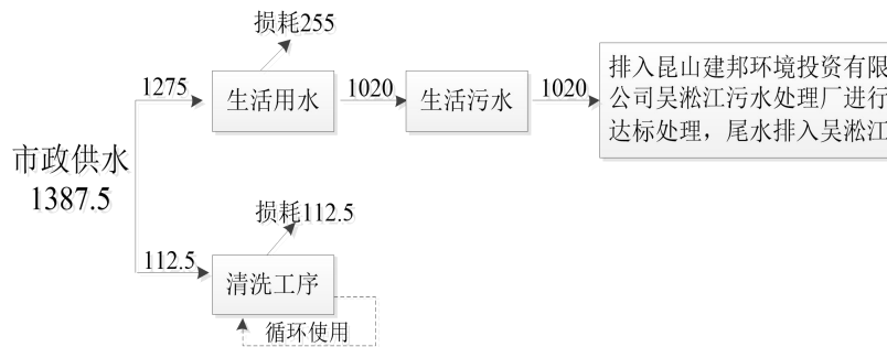
图 2-2 全厂水平衡图 (t/a)
