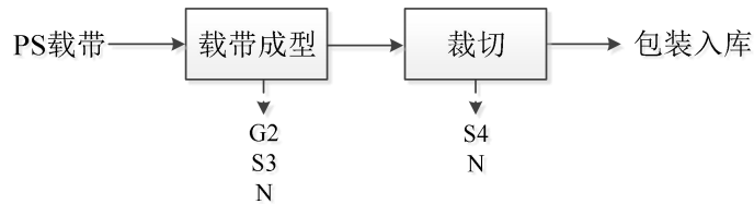
图 2-3 载带包材生产工艺流程图
