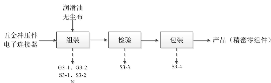
图 2-5 精密零组件生产工艺流程图
