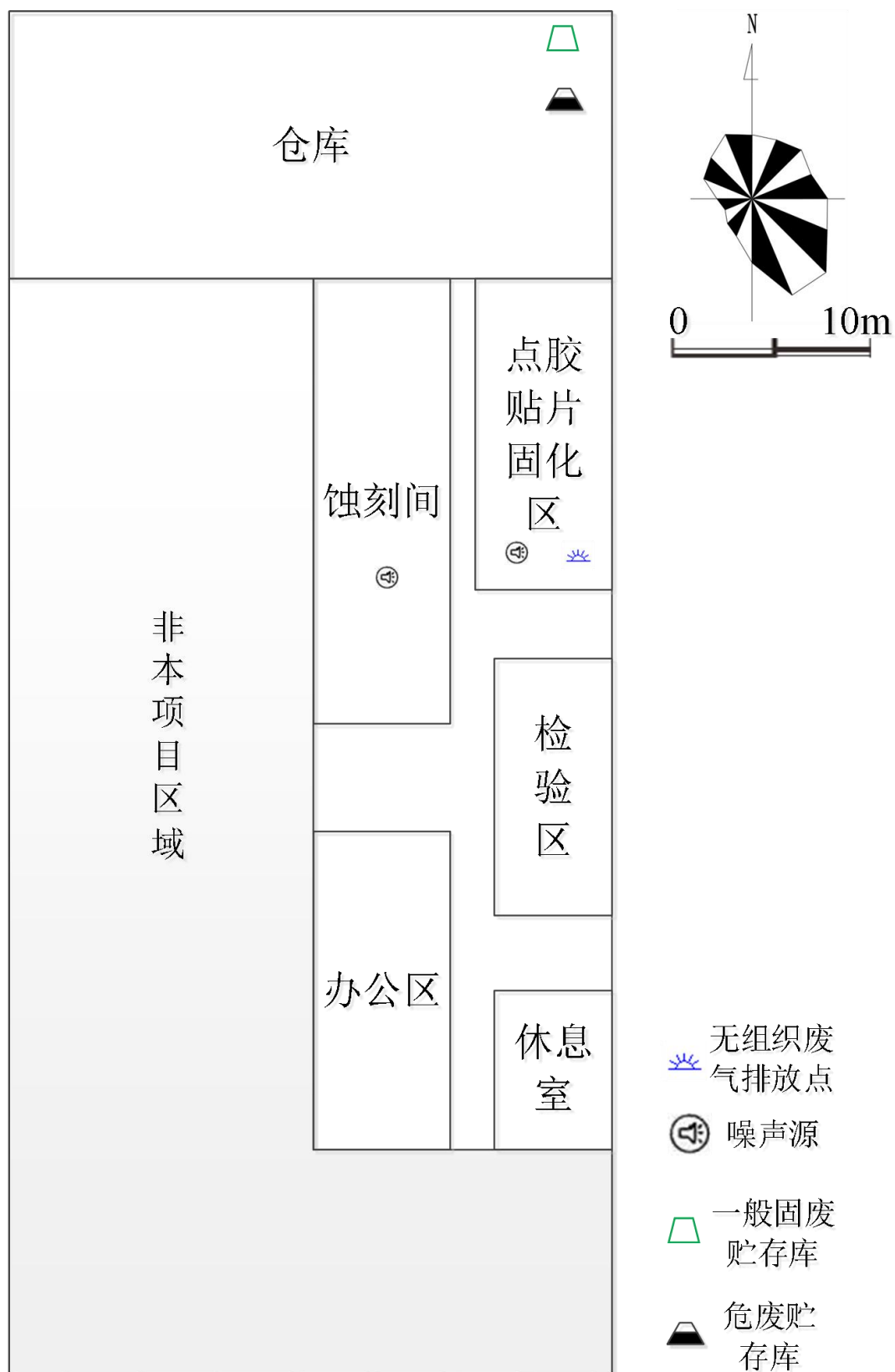
附图 4-2 项目车间内平面布置图
