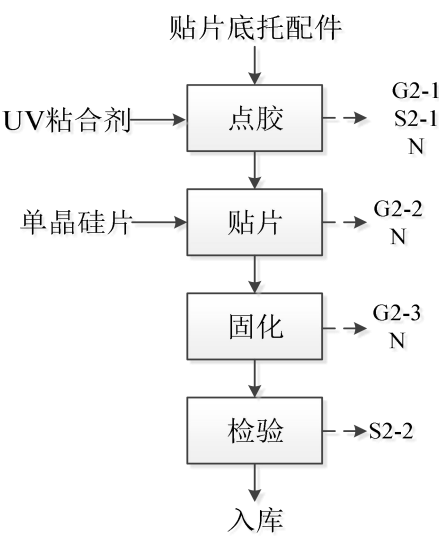
图 2-3 点胶固化工艺流程图
