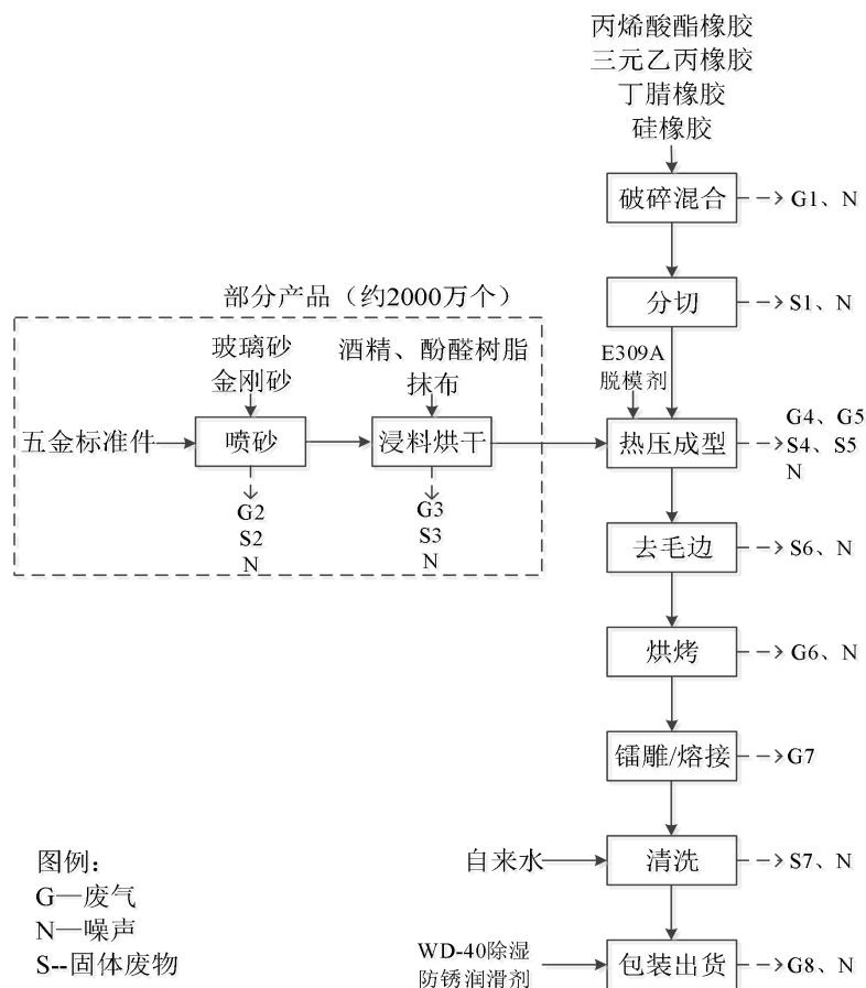
图 2-3 密封垫片生产工艺流程图
