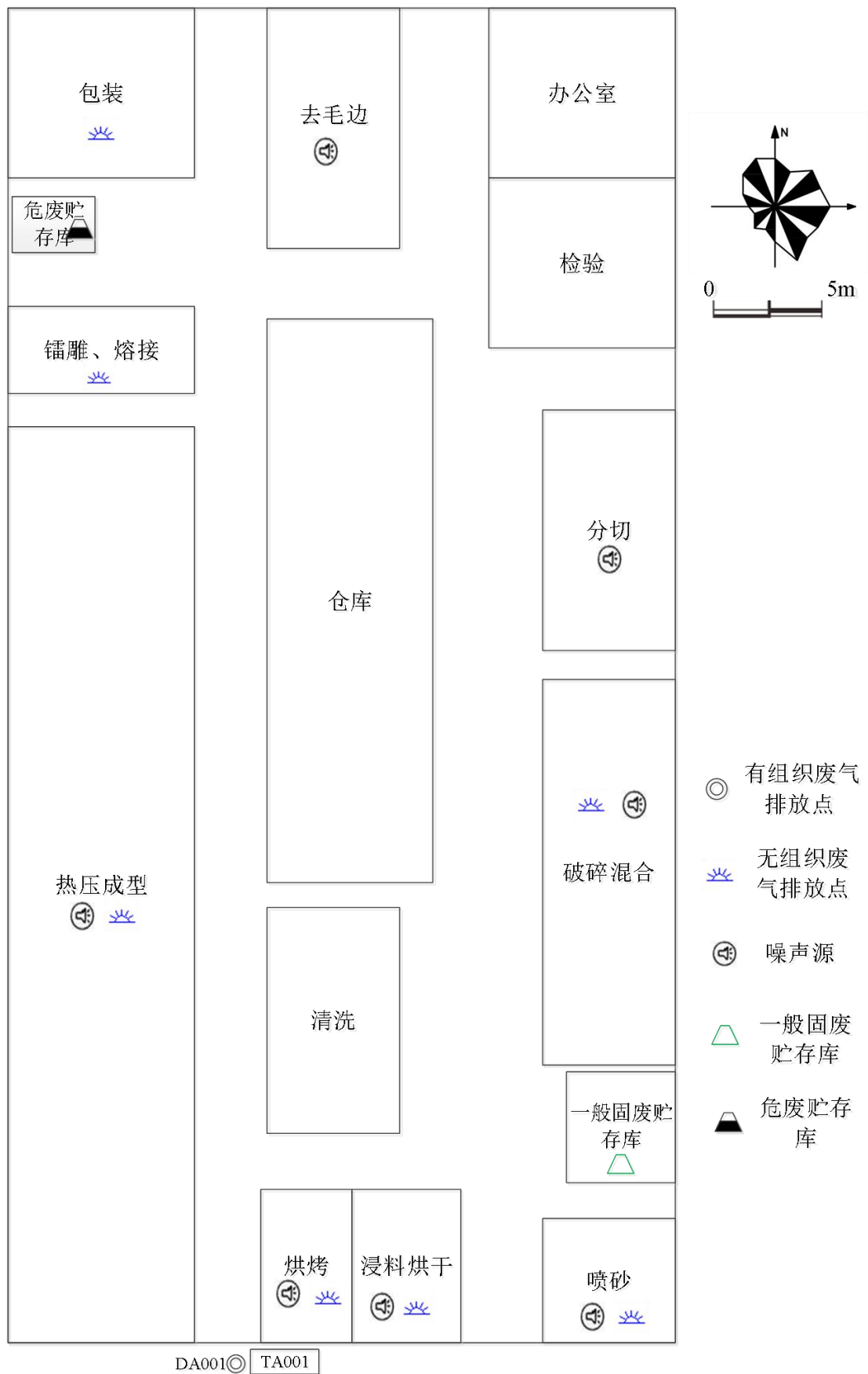
附图 4-2 项目车间内平面布置图
