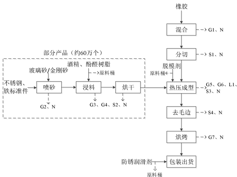
图 2-4 原有项目生产工艺流程图
