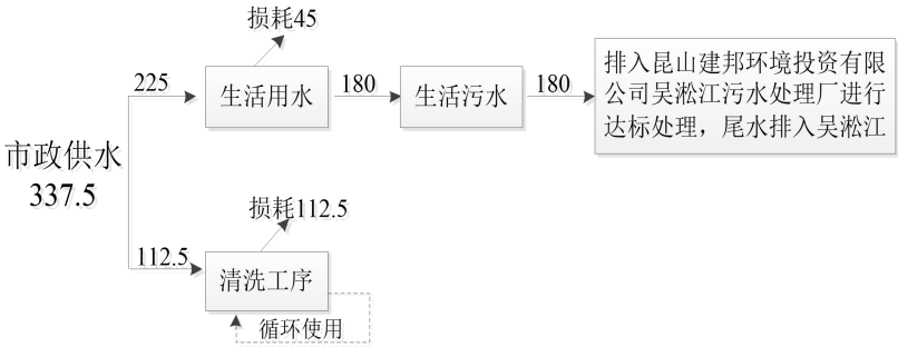
图 2-1 扩建项目水平衡图 (t/a)
