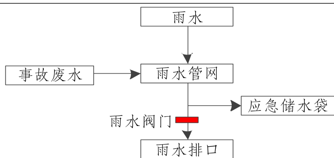
图 4-3 企业厂区事故废水收集、封堵系统示意图
