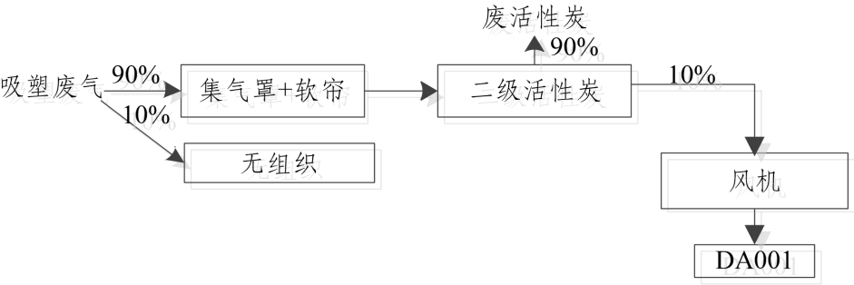
图 4-1 废气收集、处理系统图
